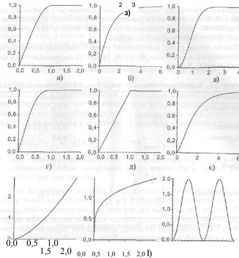
Рис. 8.5. Теоретичні варіограмні моделі при c_0 = 0 і \hat{c} = 1,0 : а) сферична; б) експоненціальна; в) гауссівська; г) пентасферична; д) лінійна; доповнена порогом; е) Бесселя; ж) степенева ( a = 1,5 ); з) степенева ( a = 0,25 ); і) періодична
